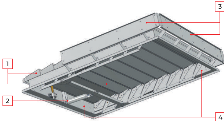
Fig. 1 Louvered vent
