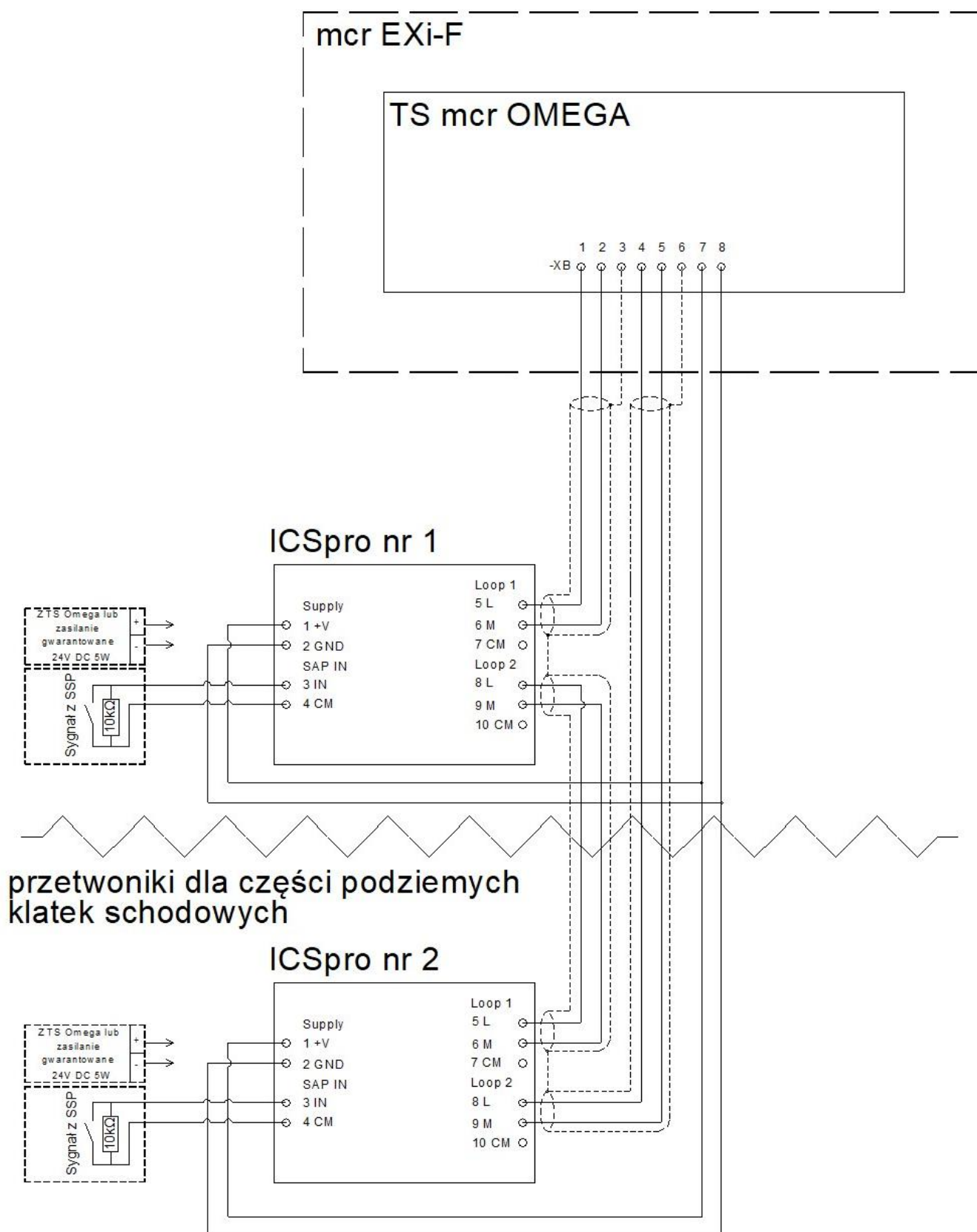
Rysunek 53. Schemat blokowy podłączeń przetworników cieśnina mcr ICSPro w układzie klatki schodowej z wydzielonymi przetwornikami w części podziemnej wzbudzanych przez SSP.
