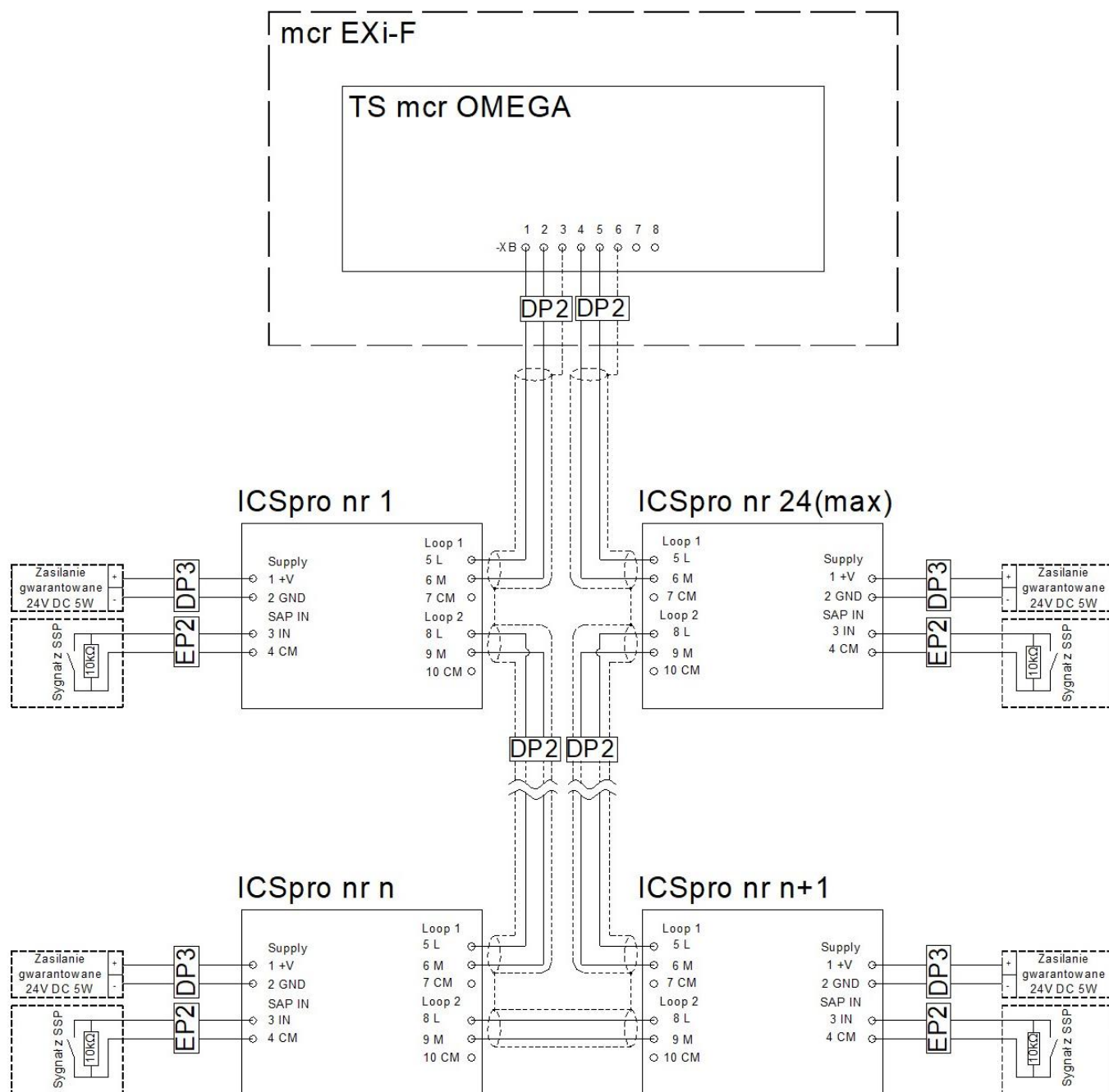
Rysunek 54. Schemat blokowy podłączeń przetworników ciśnienia mcr ICS Pro w układzie przedsionkowym.
