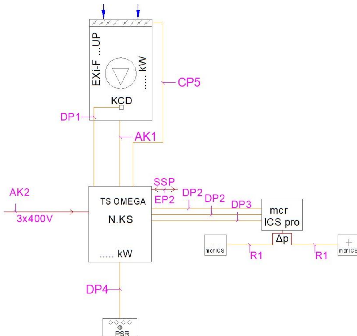
Rysunek 46. Schemat ideowy jednostki pionowej z klapą mcr LAM.
