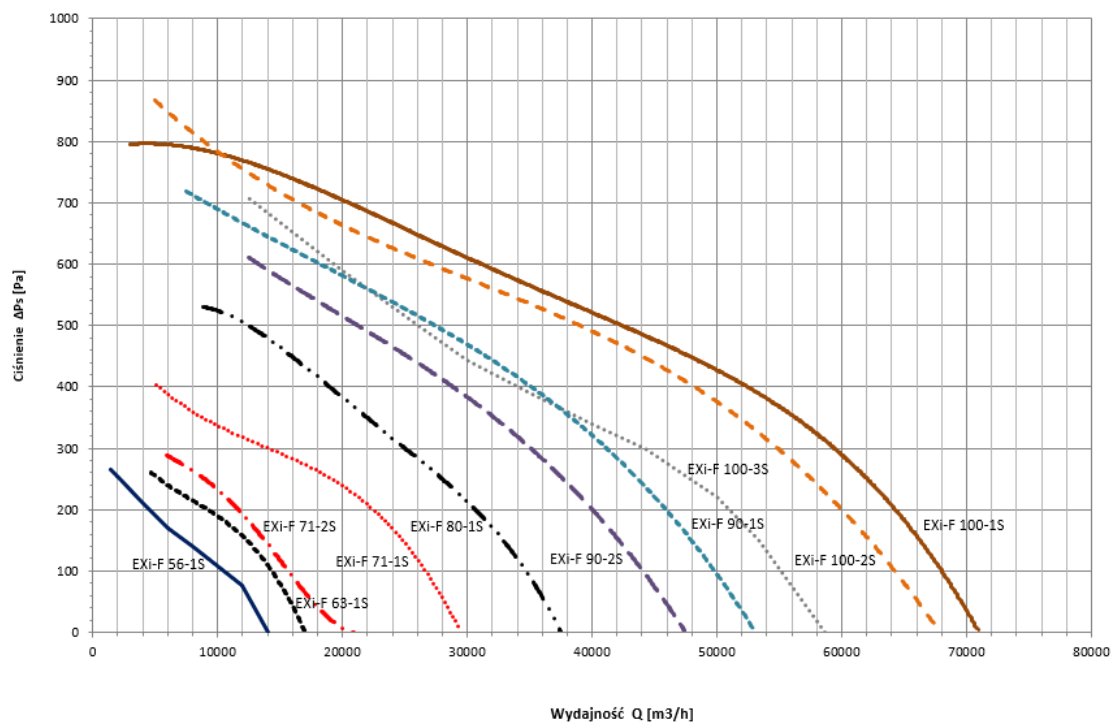
Rysunek 12. Charakterystyki urządzeń EXi-F w wariancie standardowym.
