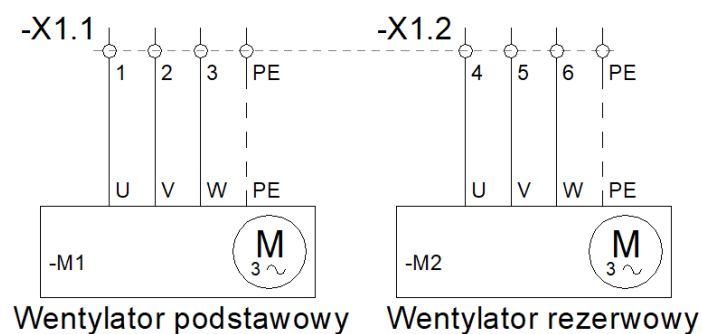
Rysunek 64. Schemat elektryczny podłączeń wentylatorów.
