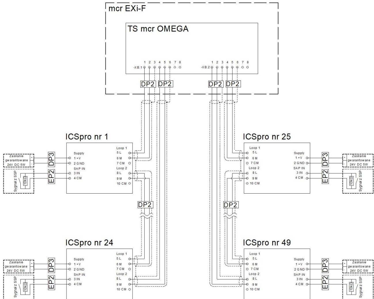
Rysunek 55. Schemat blokowy podłączeń przetworników ciśnienia mcr ICSPro w układzie przedsionkowym łączonych w dwóch pętłach komunikacji.
