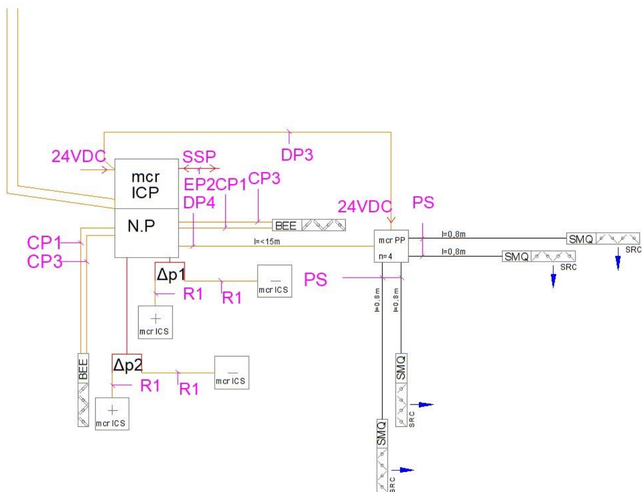
Rysunek 50. Schemat ideowy podłączenia do regulatora szybkich przepustnic mcr ICP czterech szybkich przepustnic przez puszkę mcr PP.
