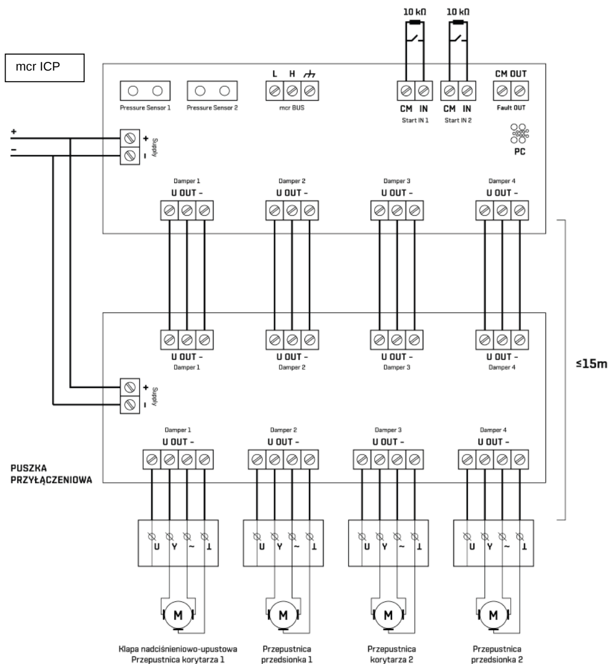
Rysunek 69. Ogólny schemat blokowy podłączeń regulatora (obsługa 4 przepustnic przedimensionowanych) mcr ICP oraz mcr PP.
