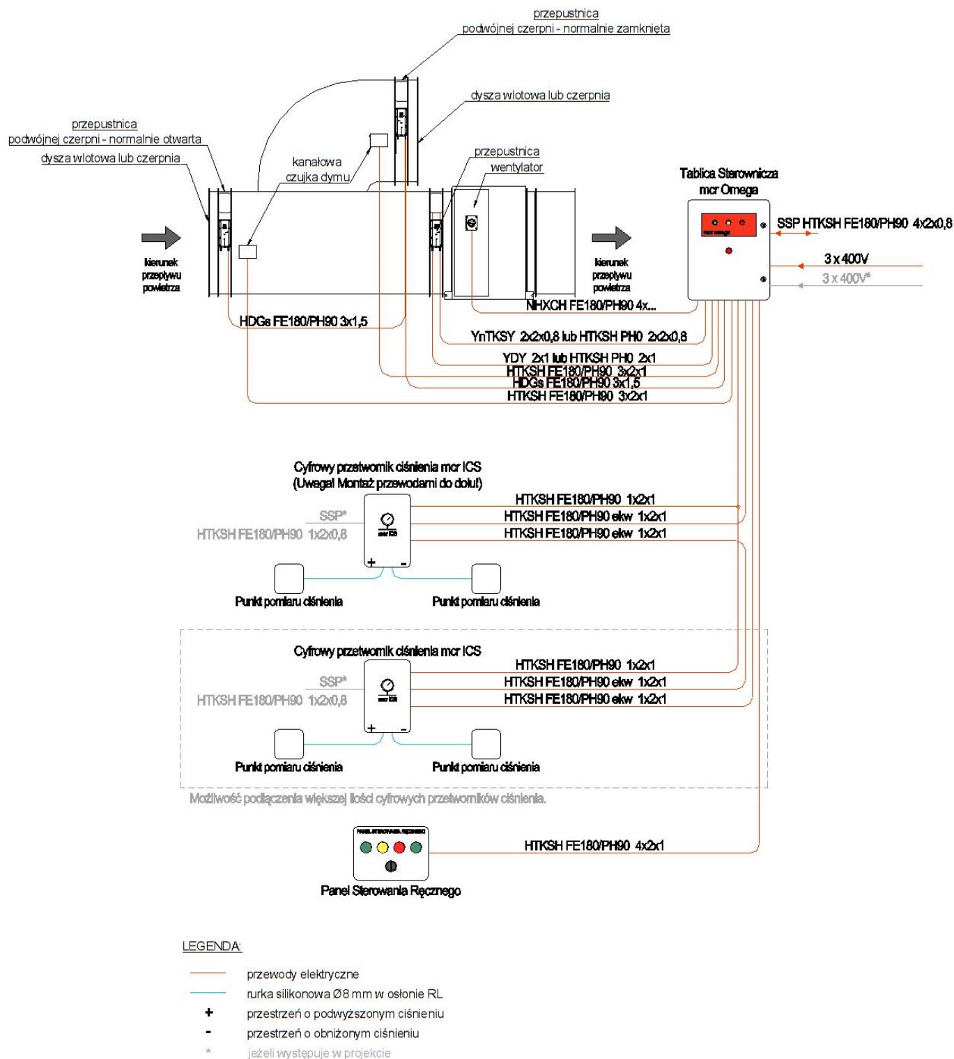
Rysunek 41. Okablowanie jednostki EXi-F z układem dwóch pompki.
