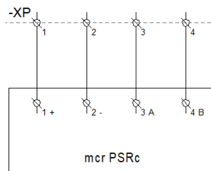
Rysunek 75. Schemat elektryczny podłączeń panelu sterowania ręcznego mcr PSRC.
