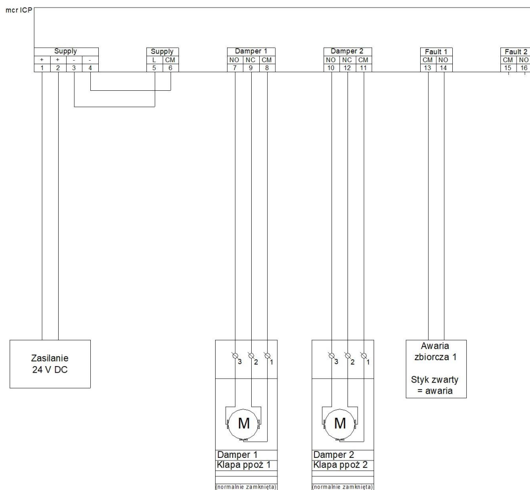
Rysunek 71. Schemat blokowy podłączeń regulatora mcr ICP – opcja z obsługą kłap wentylacji pożarowej.
