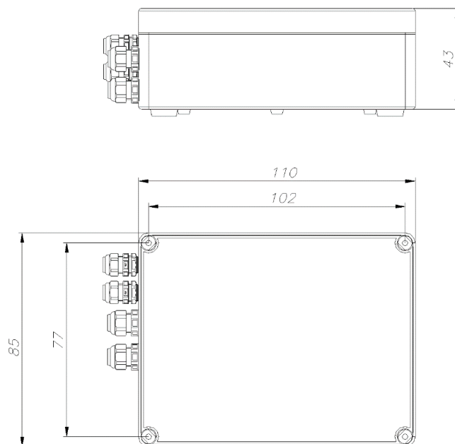
Rysunek 100. Wymiary otworów montażowych separatora sieci mcr SEP.
