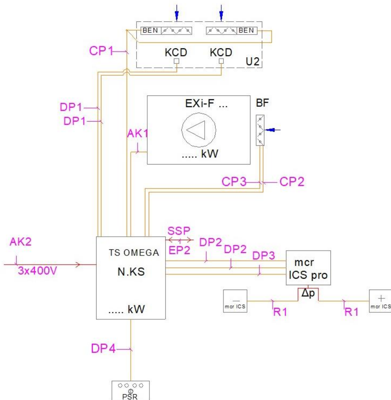
Rysunek 43. Schemat ideowy okablowania jednostki podstawowej z układem dwóch czerpni.
