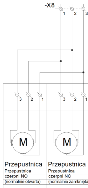
Rysunek 68. Schemat elektryczny połączeń dwóch przepustnic układu przełączania czerpni.
