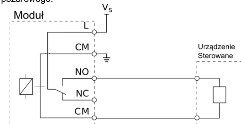
Rys. 43. Schemat połączenia wyjścia przekaźnikowego w module liniowym.
