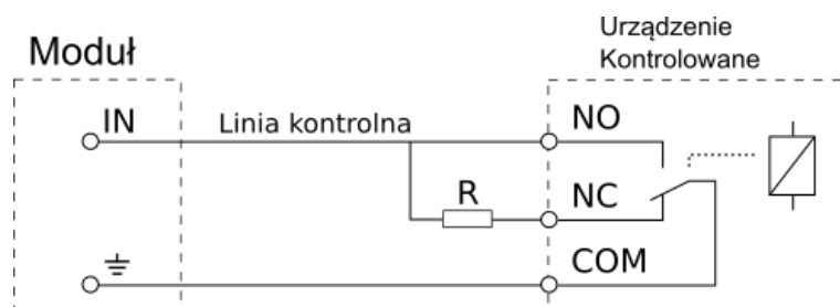
Rys. 44. Schemat podłączenia wejścia kontrolnego z kontrolą ciągłości.
