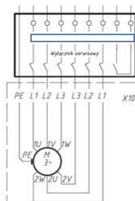
Przykładowe podłączenie wyłącznik 6-polowy
