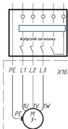
Przykładowe podłączenie - wyłącznik 3-polowy
