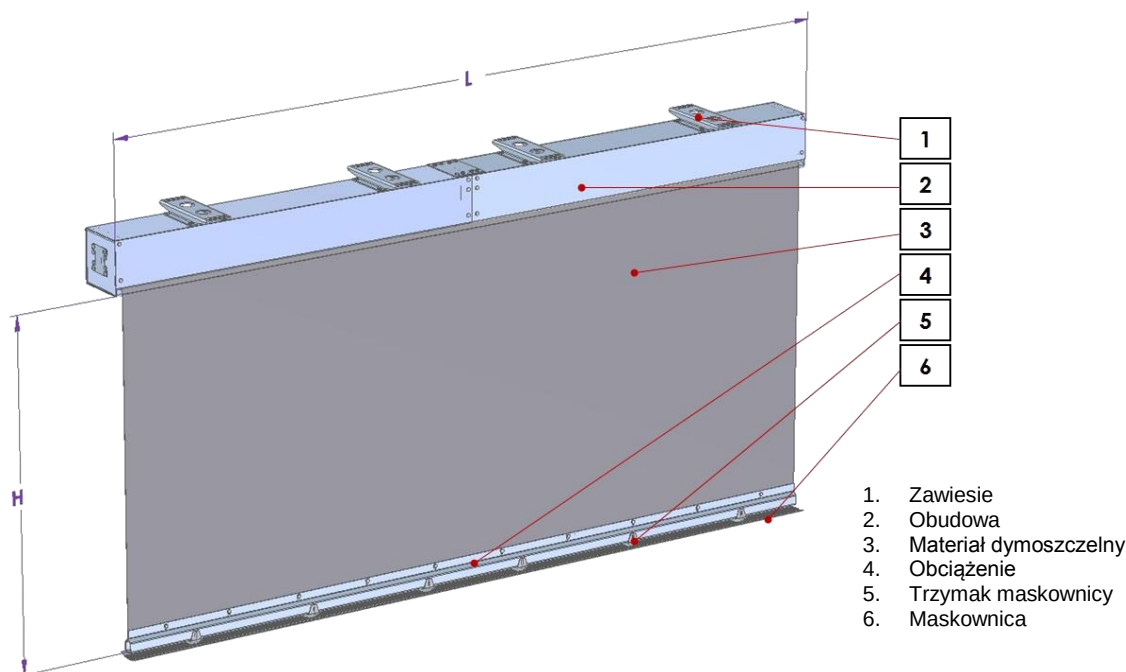
Rys. 1. Budowa rolowanej kurtyny dymowej mcr PROSMOKE FS CE .
