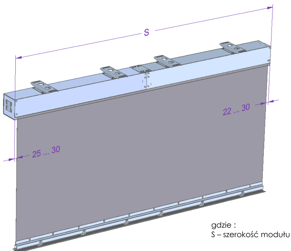
Rys.20. Wielkości szczelin w kierunku wzdłużnym kurtyn mcr PROSMOKE FS CE.
