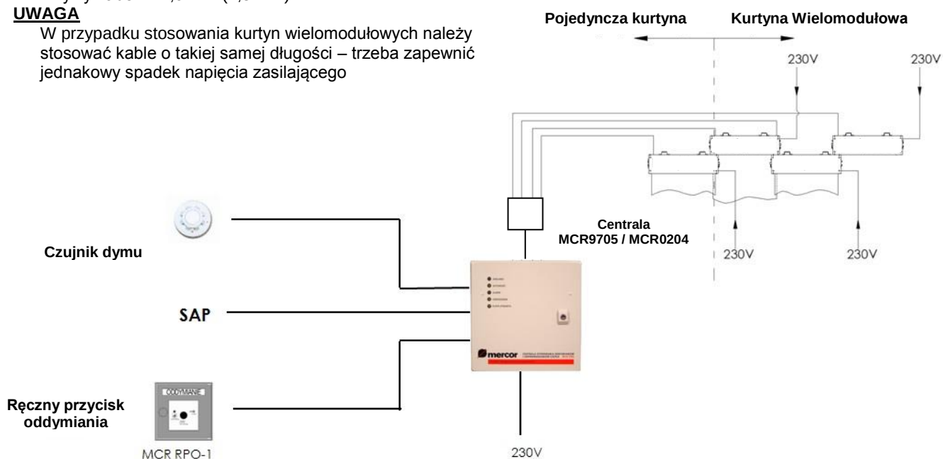
Rys.10. Schemat ideowy połączeń kurtyny ze wspólnym obciążeniem
