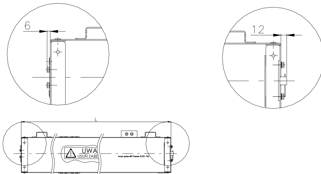
Rys. 1.1. Długości elementów wystających z obudowy kurtyn mcr PROSMOKE FS CE.
