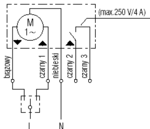
Rys. 17 Schemat podłączenia siłownik typu JMBB-500-300-LA.
