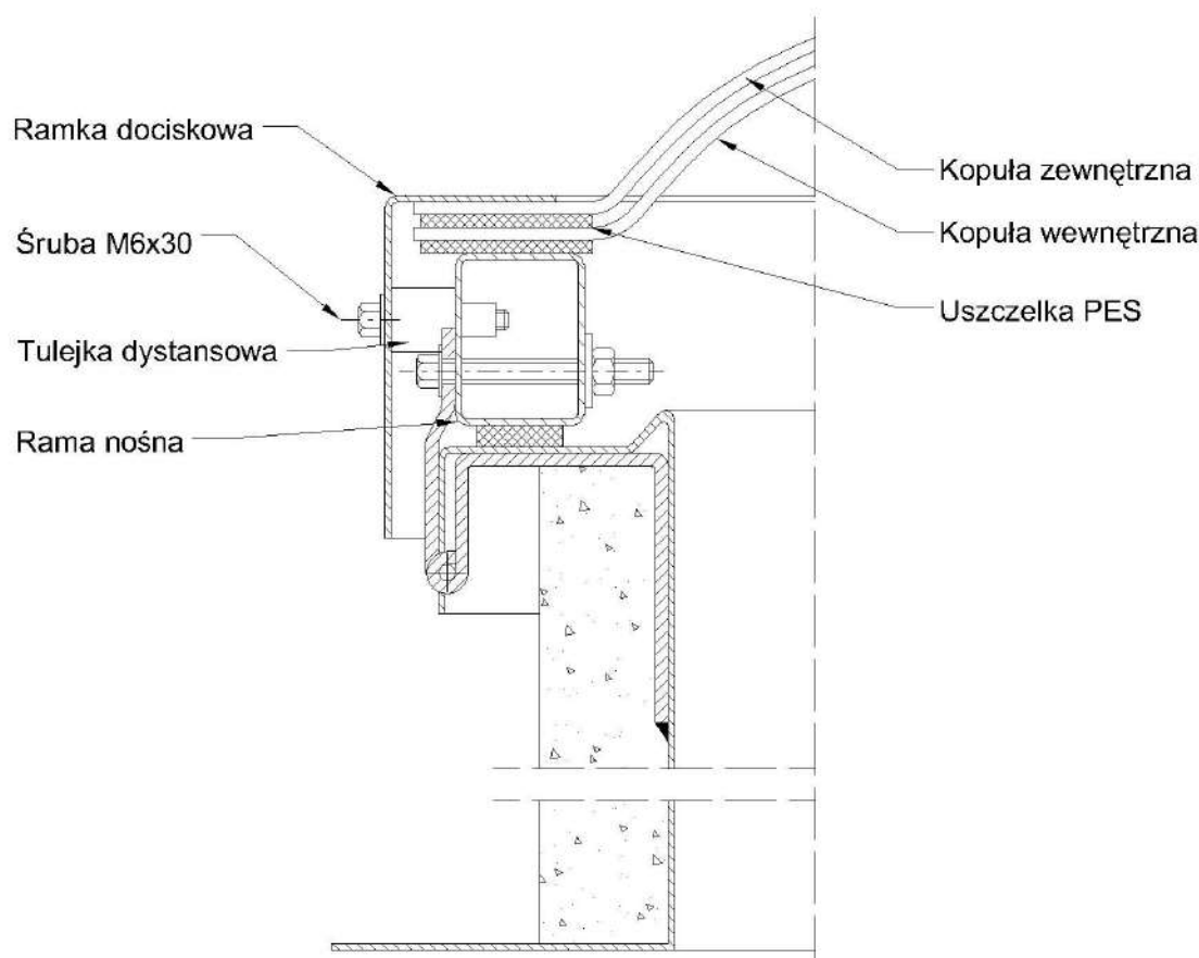
Rys. 22 Schemat zamontowanej kopuły.
