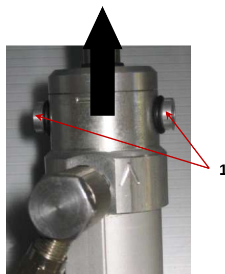
Rys. 20 Zwalnianie zamków rygla siłownika POAV.
