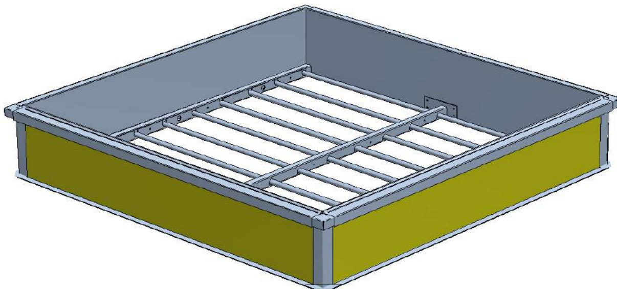
Rys. 27 Widok na podstawę świetlika stałego mcr PROLIGHT typu C z kratą antywłamaniową (widok bez wypełnienia świetlika).
