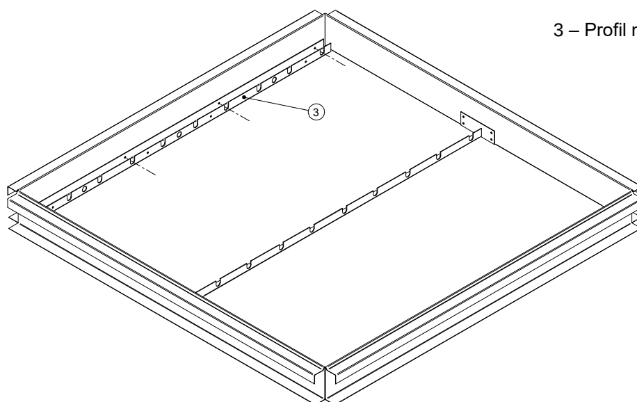
Rys. 25 Etap montażu profili nośnych kraty.
