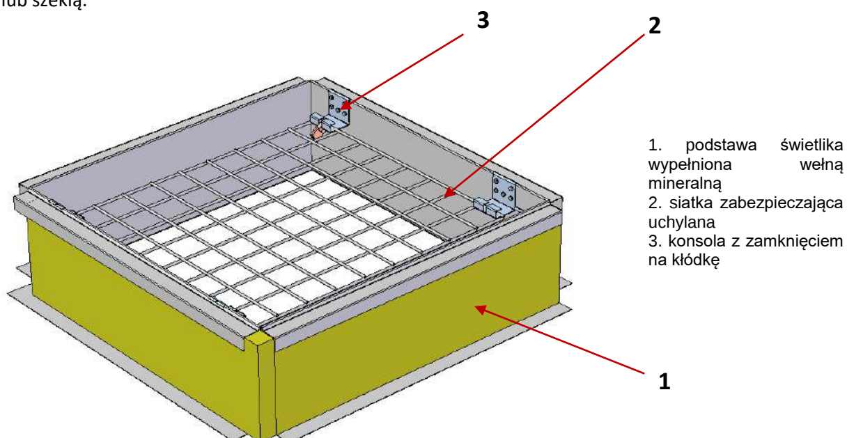
Rys. 23 Widok na podstawę świetlika otwieralnego mcr PROLIGHT typu C z uchylną siatką zabezpieczającą (bez sterowania i skrzydła świetlika).
