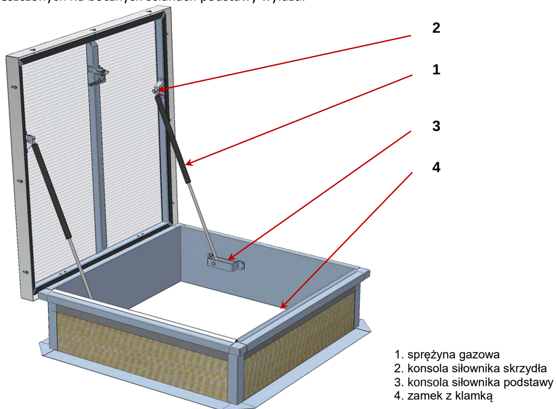
Rys. 21 Wyłaz dachowy mcr PROLIGHT typu C lub E ze sprężynami gazowymi.
