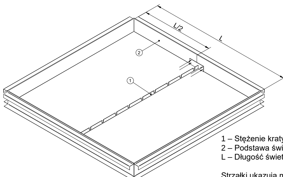
Rys. 24. Etap montażu stężenia kraty do podstawy świetlika.
