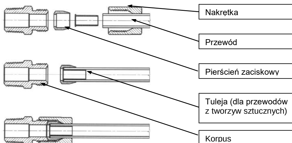
Rys. 18 Sposób montażu elastycznych przewodów instalacji pneumatycznej.
