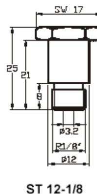
Rys. 15 Śruba ST12-1/8.
