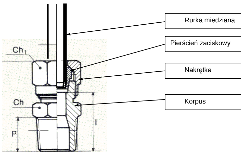
Rys. 19 Połączenie śrubunku z rurką miedzianą/stalową.
