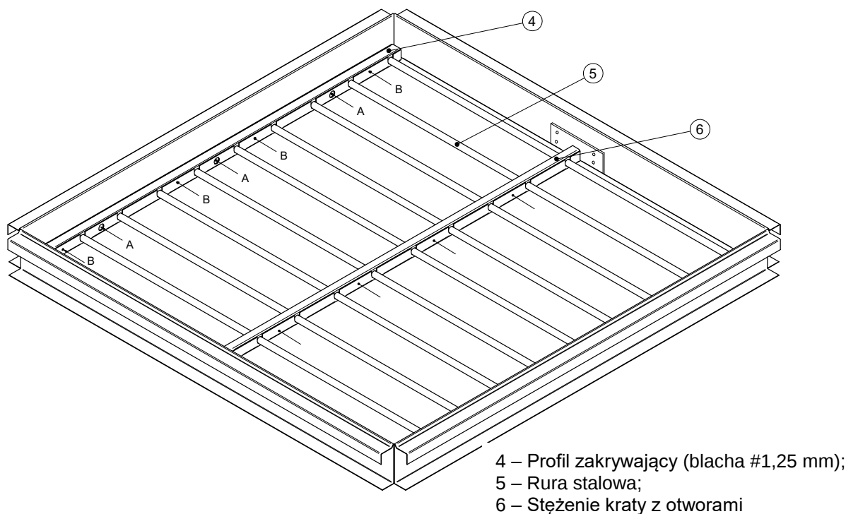
Rys. 26 Etap ułożenia rur i montażu profili zakrywających.
