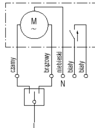
Rys. 16 Schemat podłączenia siłownika typu E-xxx-230.
