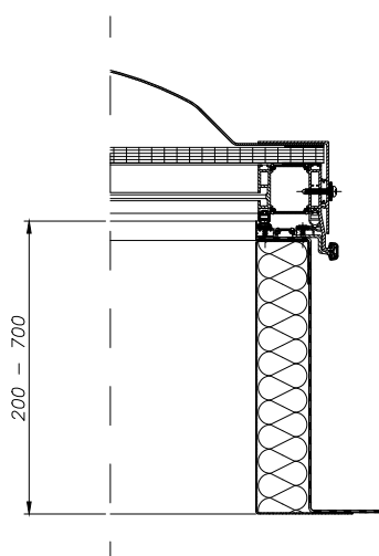
Podstawa stalowa prosta typ C/e
