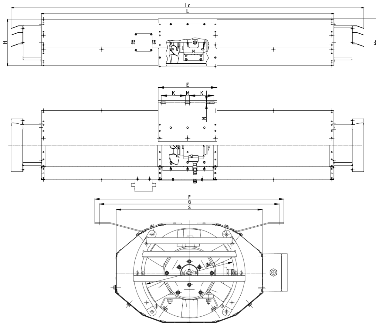
Rys 1 mcr BORA – wykonanie L lub O
