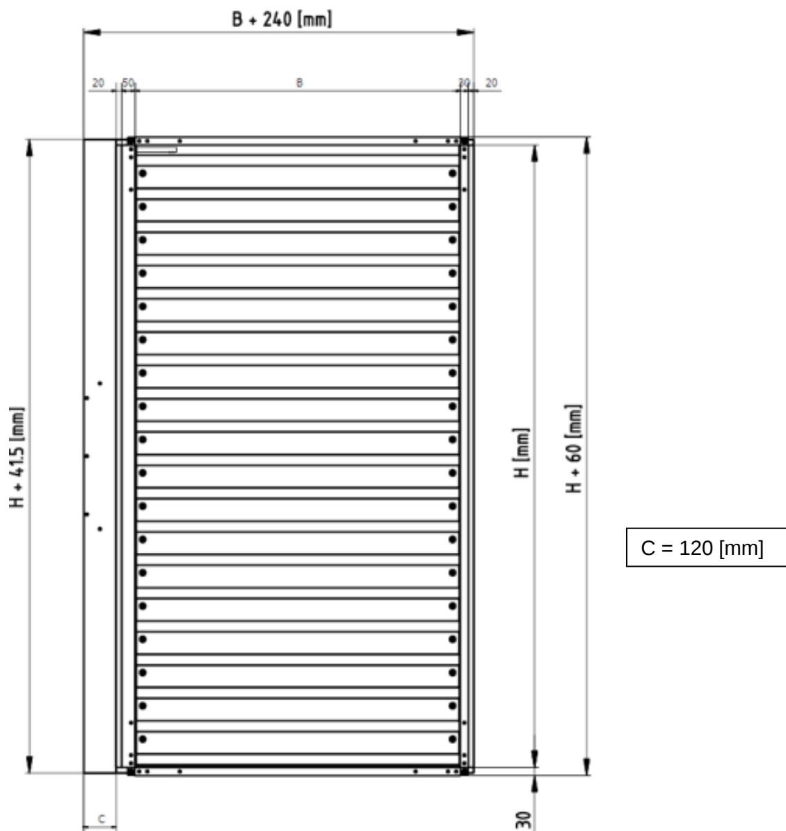
Rys. Klapa mcr WIP PROV z puszką LC mechanizmu wyzwalająco sterującego
