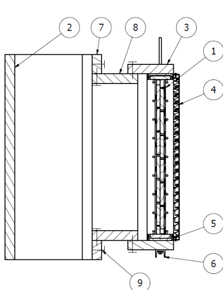
Przekrój pionowy
