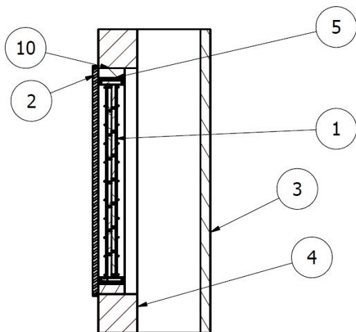
Przekrój pionowy
