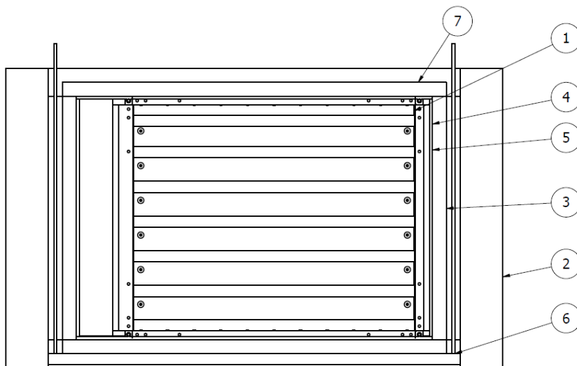
Rzut z góry –kanał pionowy
