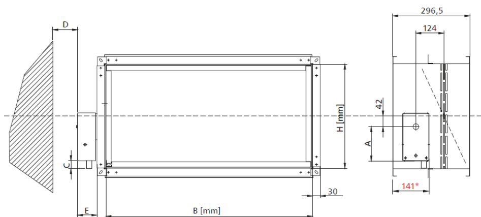
Klapa mcr FID S/... c/P z mechanizmem typu RST/KW1
