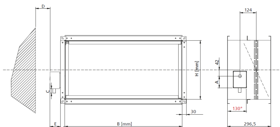
Klapa mcr FID S/... c/P z mechanizmem typu RST
