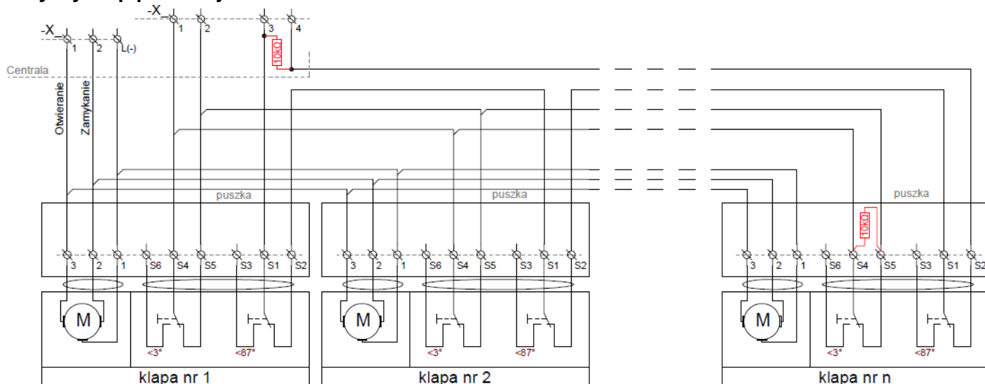
Rys. 20. Schemat siłowniki z napędem elektrycznym, normalnie zamknięte .
