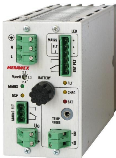
Rys. 8. Widok obudowy zasilacza.
