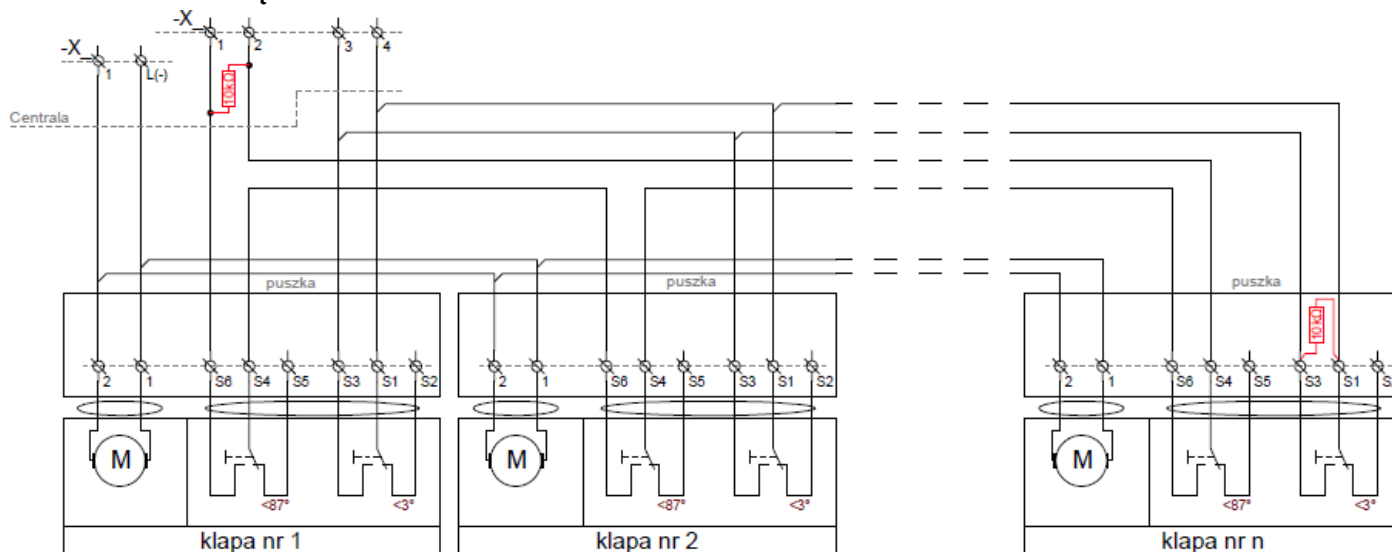
Rys. 18. Schemat siłowniki ze sprężyną otwieranie przez siłownik, normalnie zamknięte.
