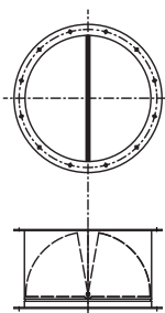
samoczynna klapa zwrotna KS-V
