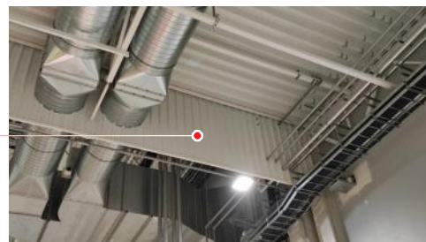
wydzielony obszar: nietypowy kształt kurtyny z połączeniami kątowymi
